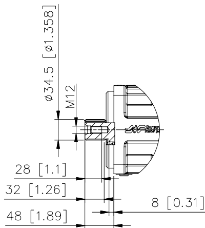
SAM SCANALATO / SPLINED W35x2x30x16 - DIN 5480
