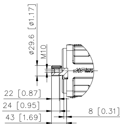
SAI SCANALATO / SPLINED W30x2x30x14 - DIN 5480
